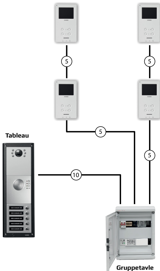
Blokdiagram
